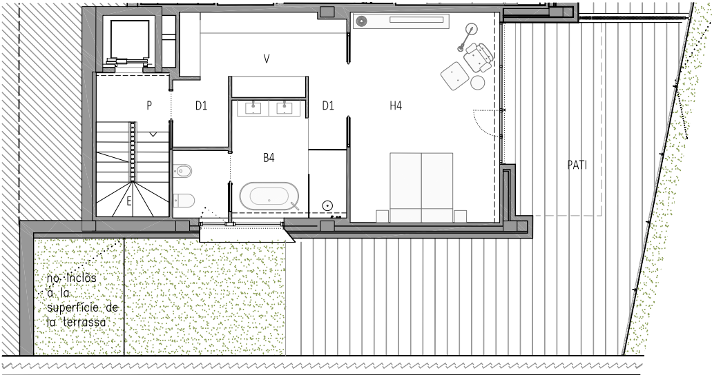
PLANTA BAIXA
